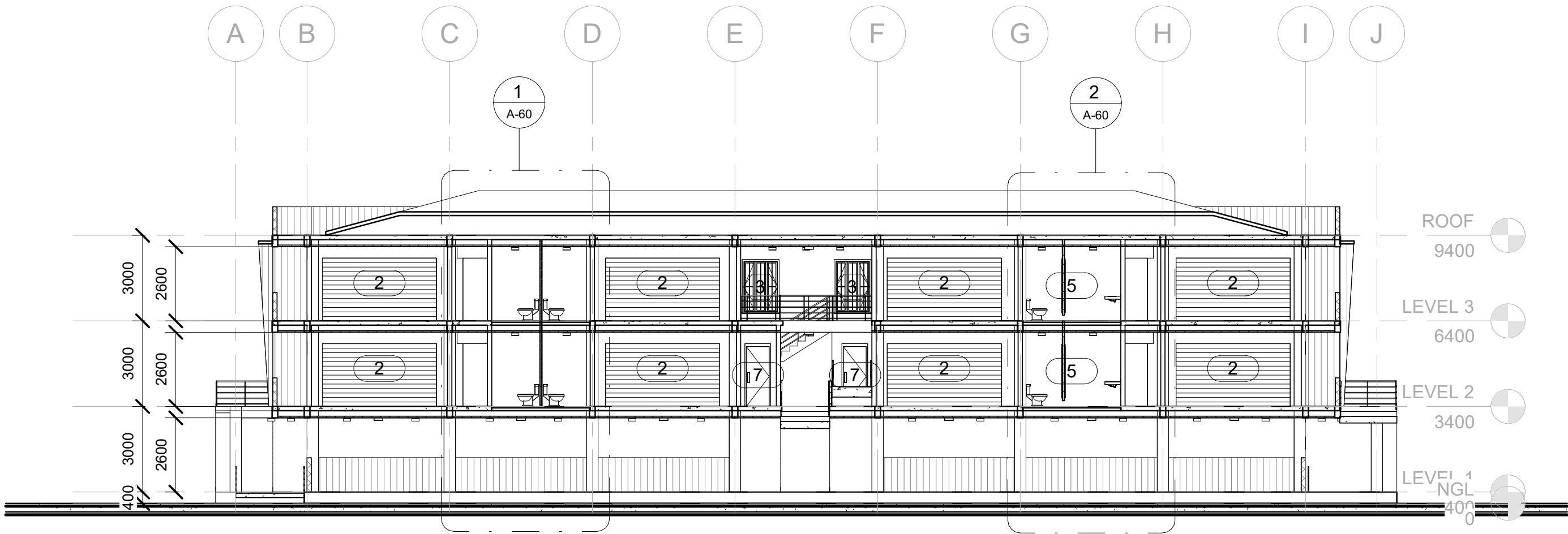
1 LONGITUDINAL SECTION 1 : 150
