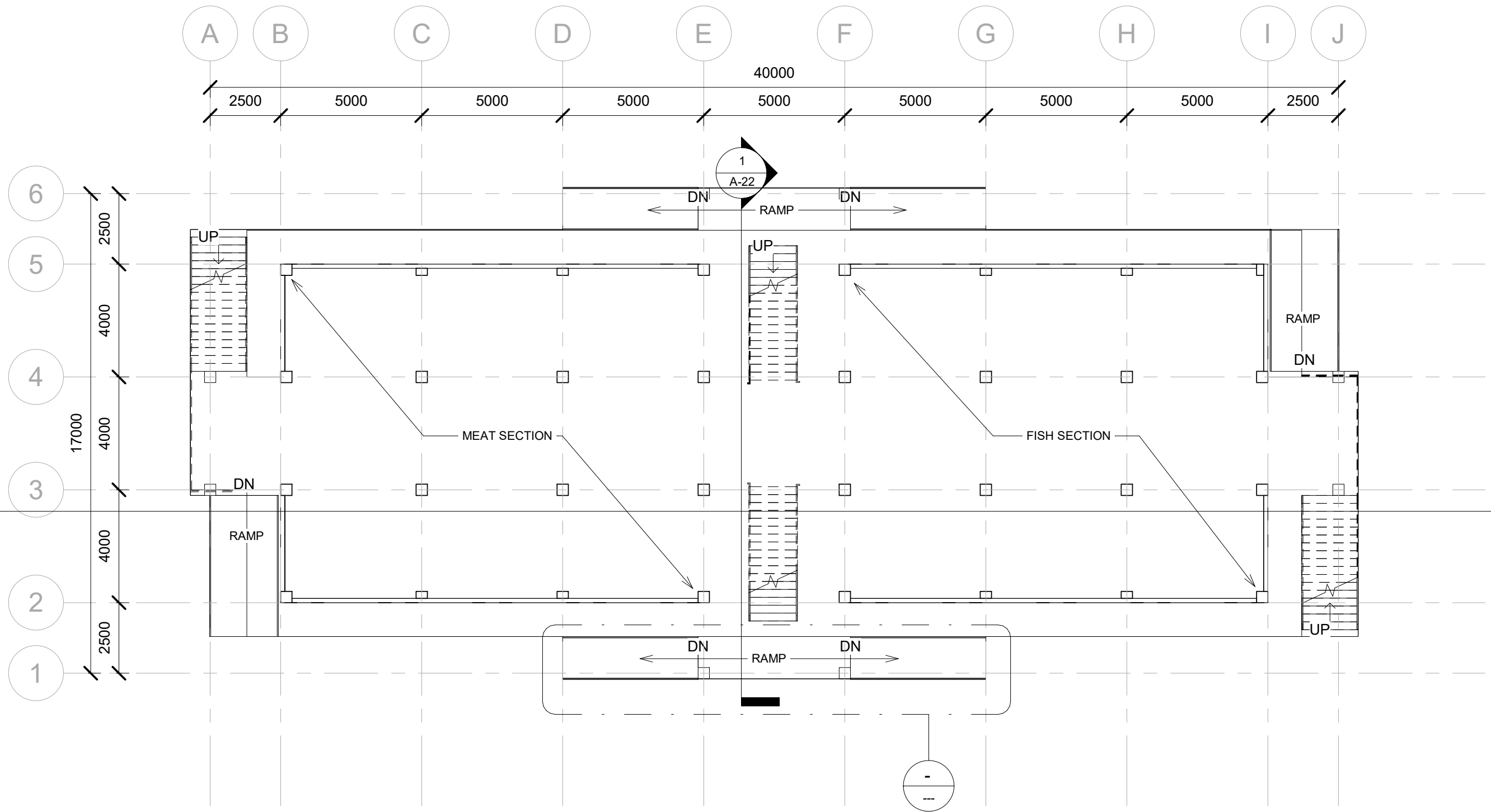
1 LEVEL 1 1 : 150
